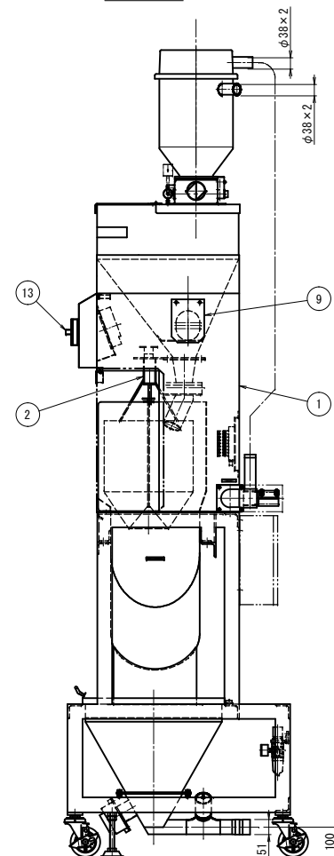
Cross section A-A A-A 断面
